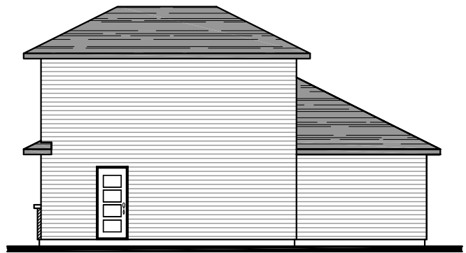
ELEVATION DROITE
